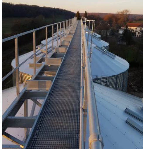
silo de stockage de Fontenois les Montbozon
